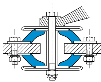
防反弹装置 (预应力)
