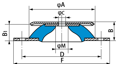
截面 XX'
