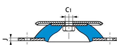
截面 XX'
