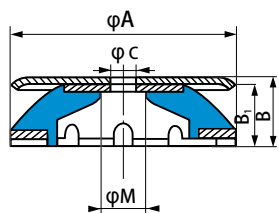
截面 XX'
