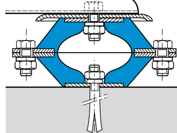
两件BECA底座的安装 (双倍的形变量)
